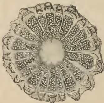
Fig. 7. - Sección de junco.
